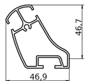
BOTTOM BAR
